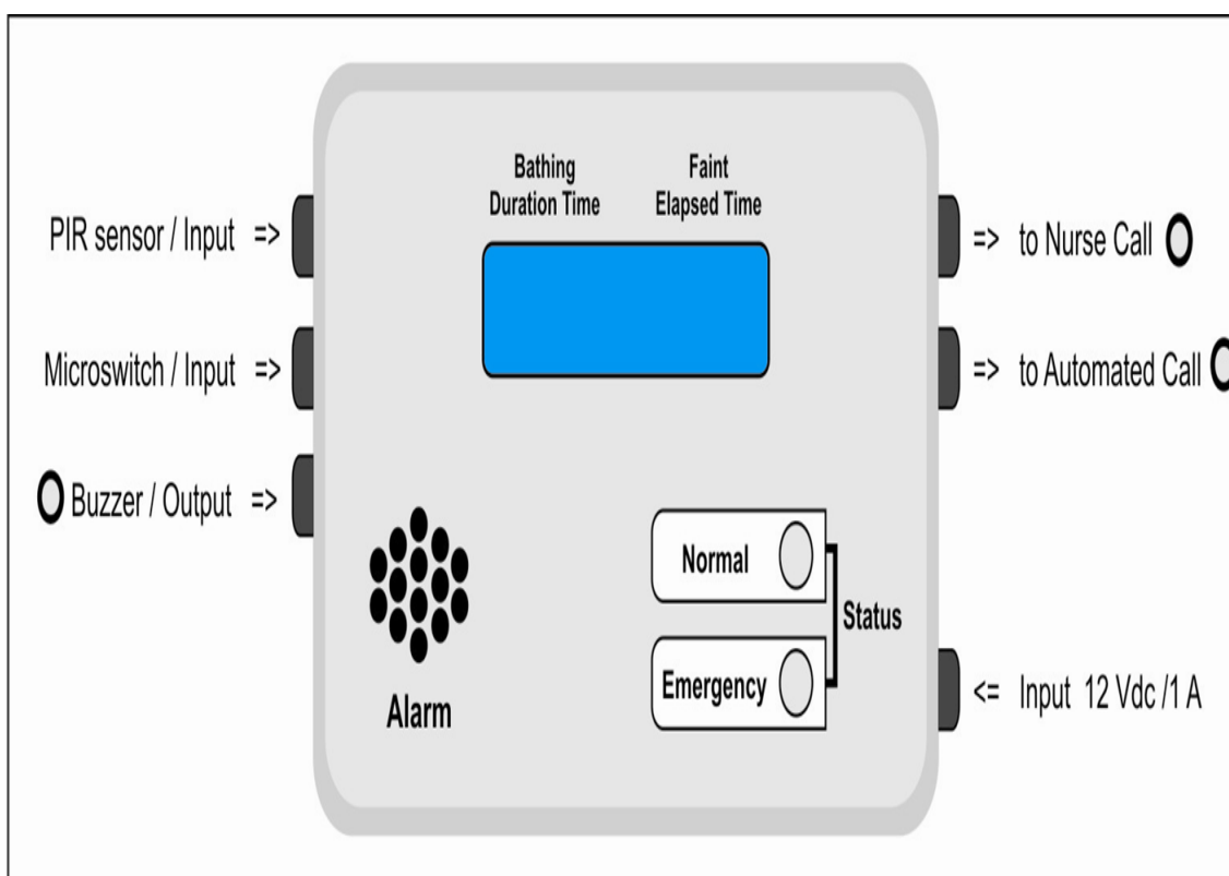
شکل ۱- دستگاه تشخیص‌دهنده غش در حمام (پردازش‌گر مرکزی)
